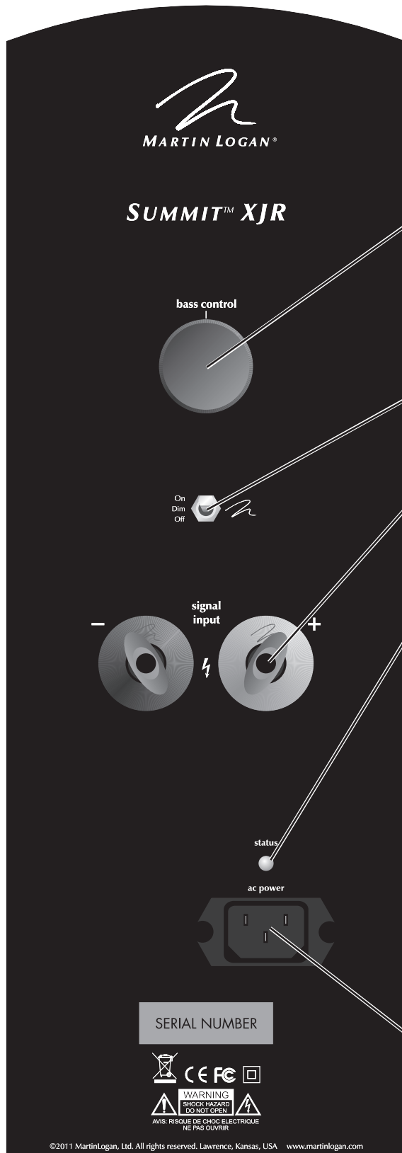
Figure 1. Raccord Summit XJR et panneau de commande.
